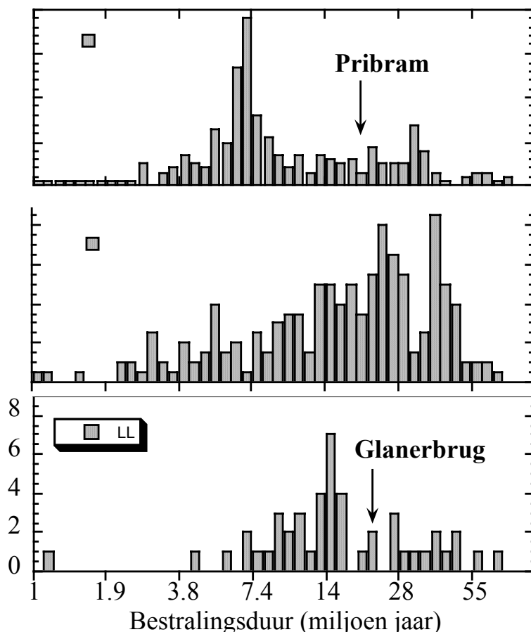
Figuur 4. Bestralingsduur van 262 H-, 218 L- en 47 LL-chondrieten, gebaseerd op ^3\text{He} , ^{21}\text{Ne} en ^{38}\text{Ar} concentraties [18]. De x-as is logaritmisch met een resolutie van 10%. De bestralingsduur van 19 miljoen jaar voor Příbram en 22 miljoen jaar voor Glanerbrug vallen niet in de voornaamste clusters van 7 miljoen jaar voor H-chondrieten en 15 miljoen jaar voor LL chondrieten.
