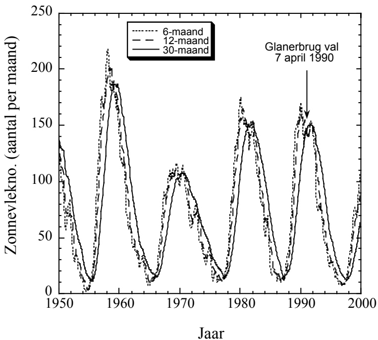
Figuur 1. Zonnevlek cyclus voor de periode 1950-2000. De drie curves tonen 6-maand, 12-maand en 30-maand gemiddelden van het aantal zonnevlekken per maand. De Glanerbrug viel halverwege het laatste maximum in de 11-jarige zonnevlek cyclus, dat duurde van 1989-1991.
