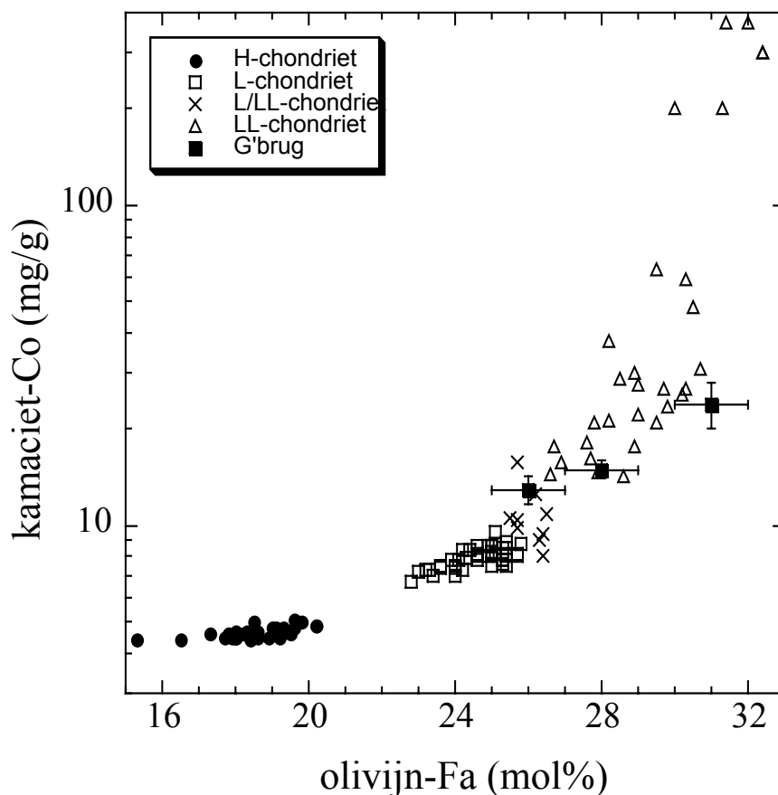
Figuur 2 : Kamaciet-Co gehalte en olivijn-fayaliet gehalte in drie fragmenten van de Glanerbrug in vergelijking met analyses aan ~120 gewone chondrieten [8]. De H-chondrieten zijn duidelijk van de L en LL-chondrieten gescheiden, maar de grens tussen L en LL chondrieten is arbitrair, zodat voorlopig ca. 10 chondrieten als L/LL worden aangeduid.
