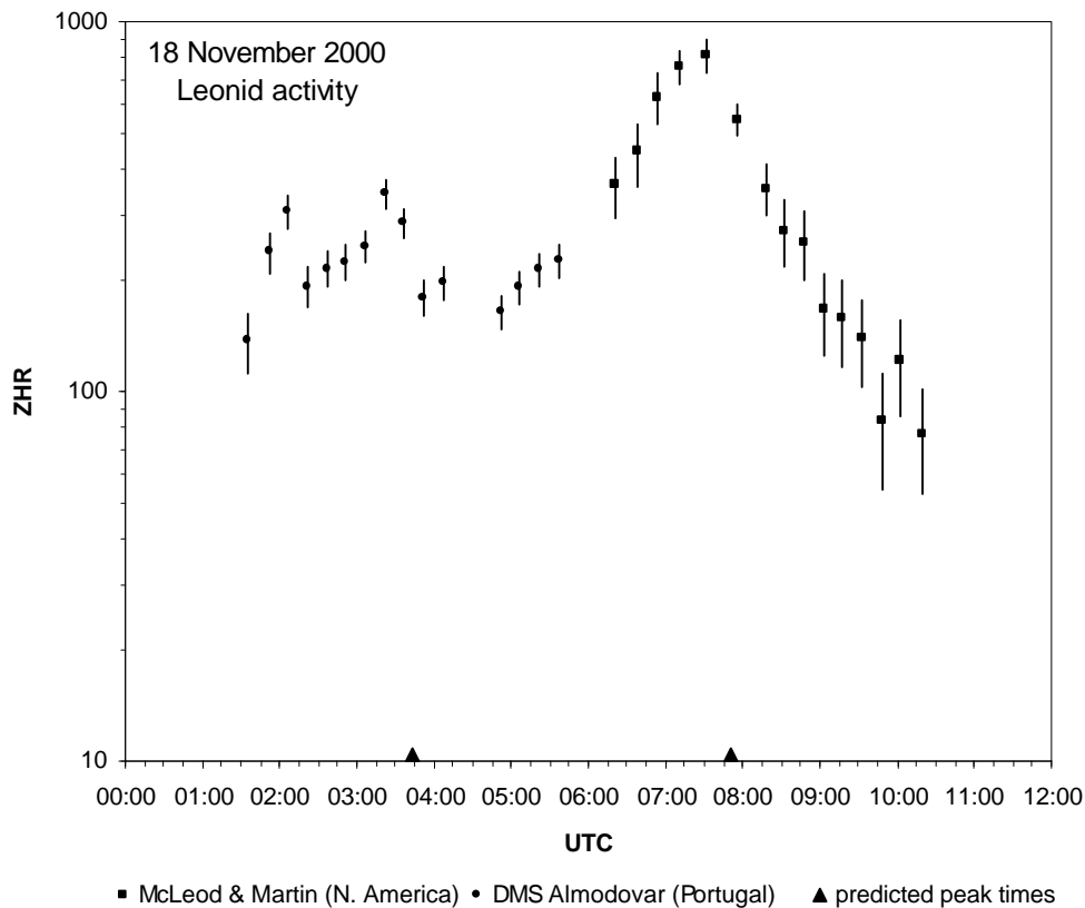
Figuur 3: De waarnemingen van het DMS team te Almodovar, Portugal (CJD, KMH, MLV) van de nacht 17-18 november gecombineerd met de waarnemingen van Pierre Martin (Quebec, Canada) en AMS waarnemer Norman McLeod III (Fort Myers, Florida, USA). Duidelijk is de forse piek boven het Amerikaanse continent met maximum ZHR ~ 800 rond 7:20 UTC en B ~11 te zien. Een eerste aanzet van deze piek is al zichtbaar in de Portugese data: de oplopende uurfrequenties in deze data en de Amerikaanse data sluiten zeer fraai op elkaar aan. Net als in figuur 1 en 2 is rekening gehouden met de perceptie van de waarnemers. Er is gerekend met een gamma-waarde van -1.4 in de radiant-hoogte-correctie. Zie ook figuur 2 voor de piek rond 3:25 UTC en de sub-piek rond 2:00 UTC.
